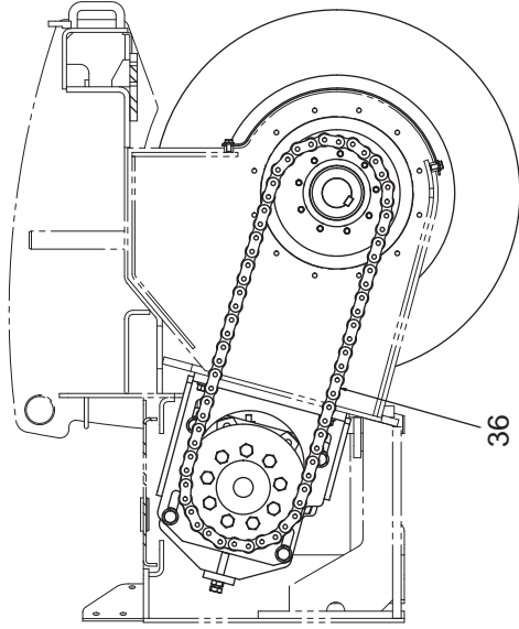
断面 B-B
