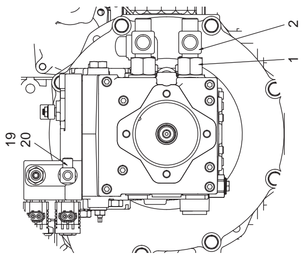
詳細 E
