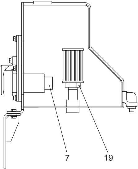
断面 A-A
