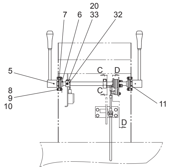
矢視 B
