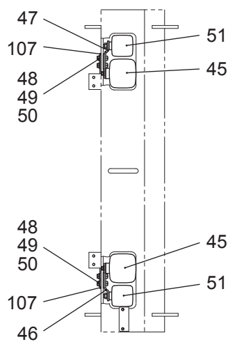
矢視 A
