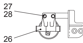
#26 燃料フィルター取付詳細
