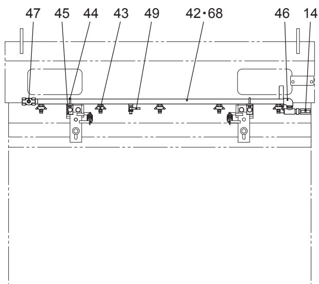
矢視 A
