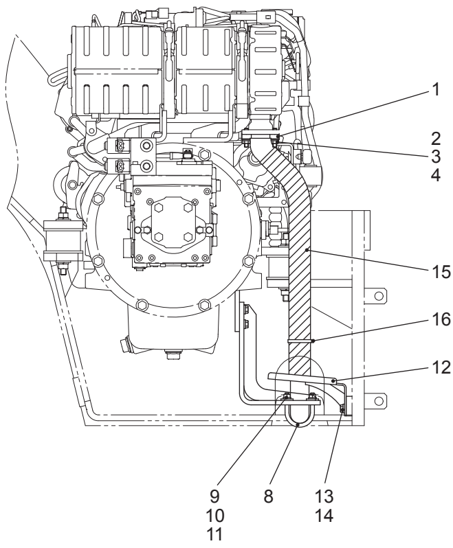
矢視 A
