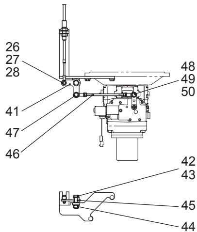
A部詳細
