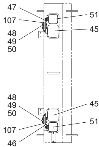
矢視 A
