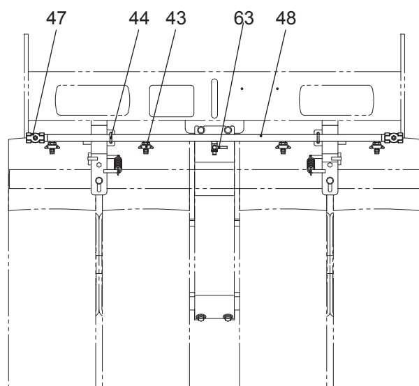
矢視 B
