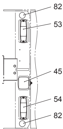
矢視 B
